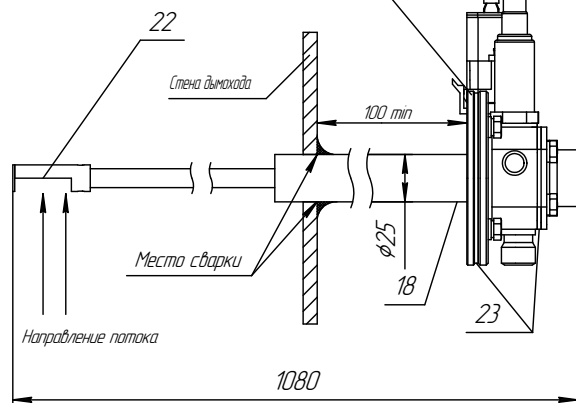
Монтаж БОП в металлическую стену
